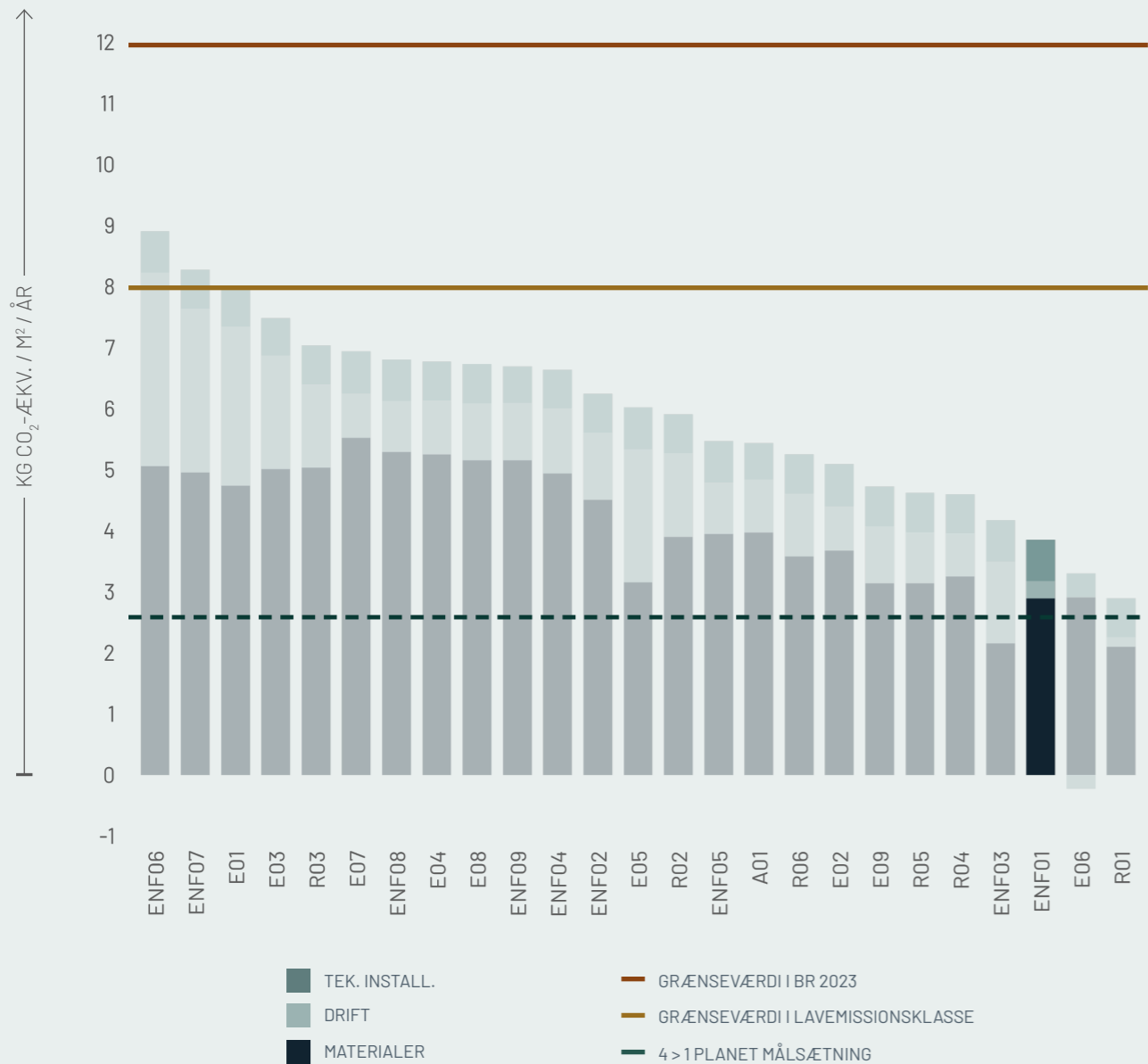
Figur ENF01.5: Boligcases
