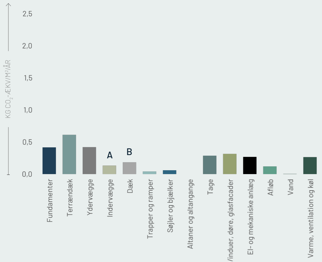
Figur E06.7: CO 2 -regnskab over byggeriets bygningsdele Den horisontale akse viser bygningens mest centrale bygningsdele, herunder fundamenter, terrændæk, ydervægge, indervægge, dæk, trapper og ramper, søjler og bjælker, altaner og altangange, tage, vinduer, døre og glasfacader, el- og mekaniske anlæg samt tekniske installationer (standard værdier).
