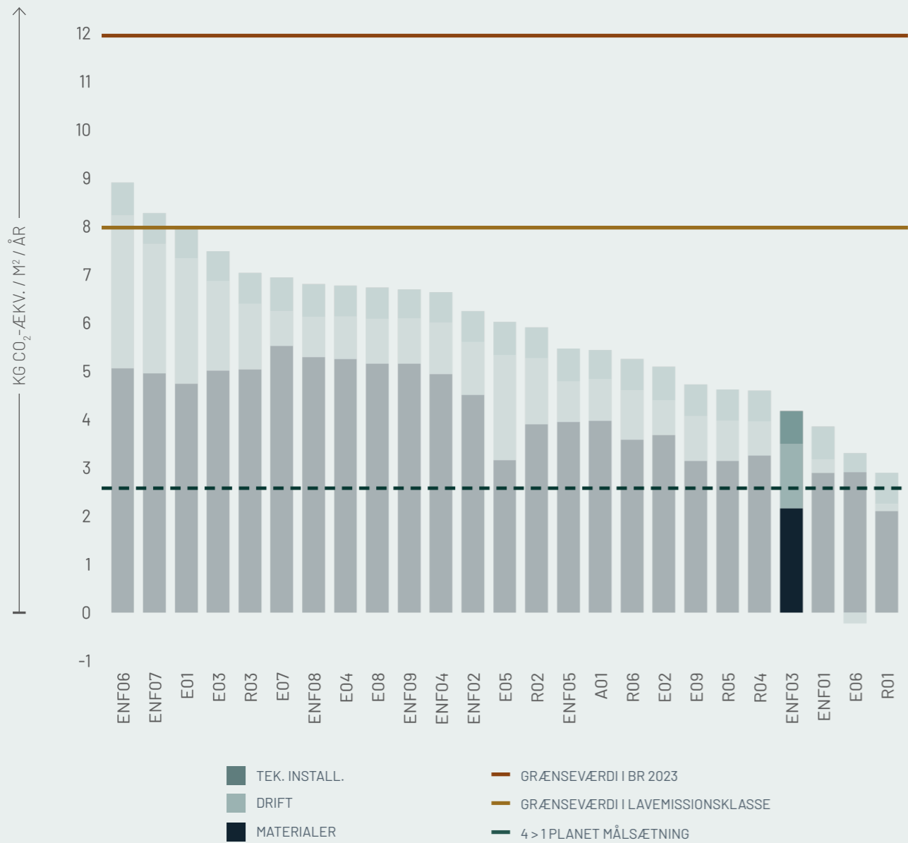
Figur ENF03.5: Boligcases Den vertikale akse viser udledning af kg CO 2 -ækv. / m 2 / år. Den horisontale akse viser de 25 best practice cases.
