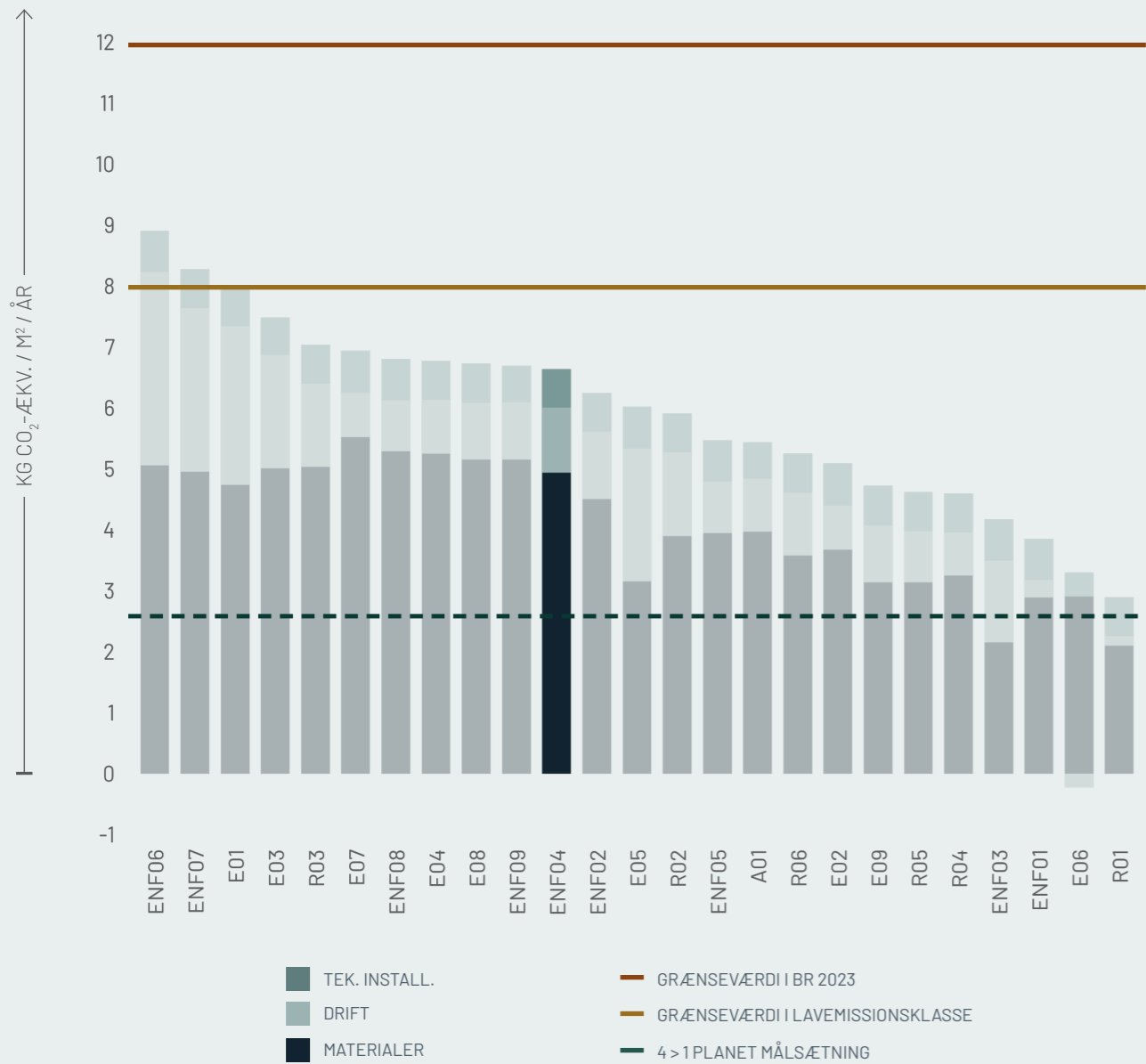
Figur ENF04.5: Boligcases Den vertikale akse viser udledning af kg CO 2 -ækv. / m 2 / år. Den horisontale akse viser de 25 best practice cases.
