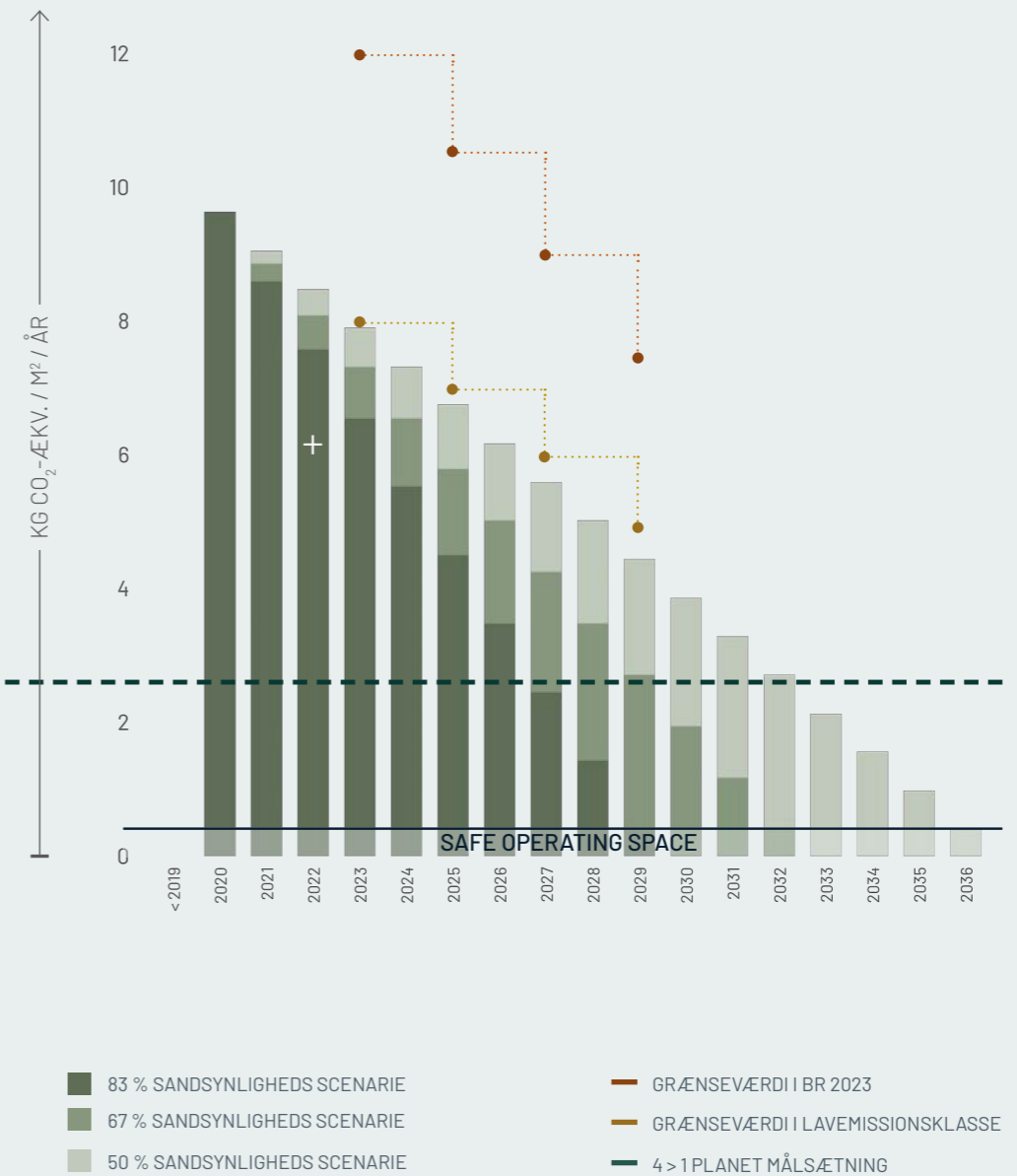
Figur E04.6: Reduction Roadmap Den aktuelle case i relation til Reduction Roadmap, grænseværdierne, 4 til 1 planets målsætning på 2.5 kg CO 2 - ækv./m 2 / år og 'safe operating space'.
