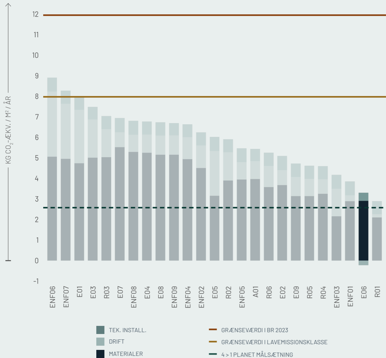
Figur E06.5: Boligcases Den vertikale akse viser udledning af kg CO 2 -ækv./m 2 /år. Den horisontale akse viser de 25 best practice cases.
