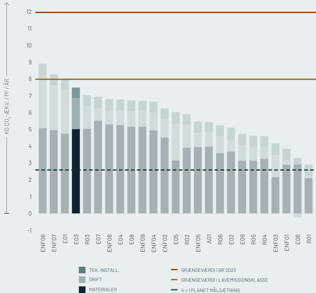
Figur E03.5: Boligcases Den vertikale akse viser udledning af kg CO 2 -ækv./m 2 /år. Den horisontale akse viser de 25 best practice cases.
