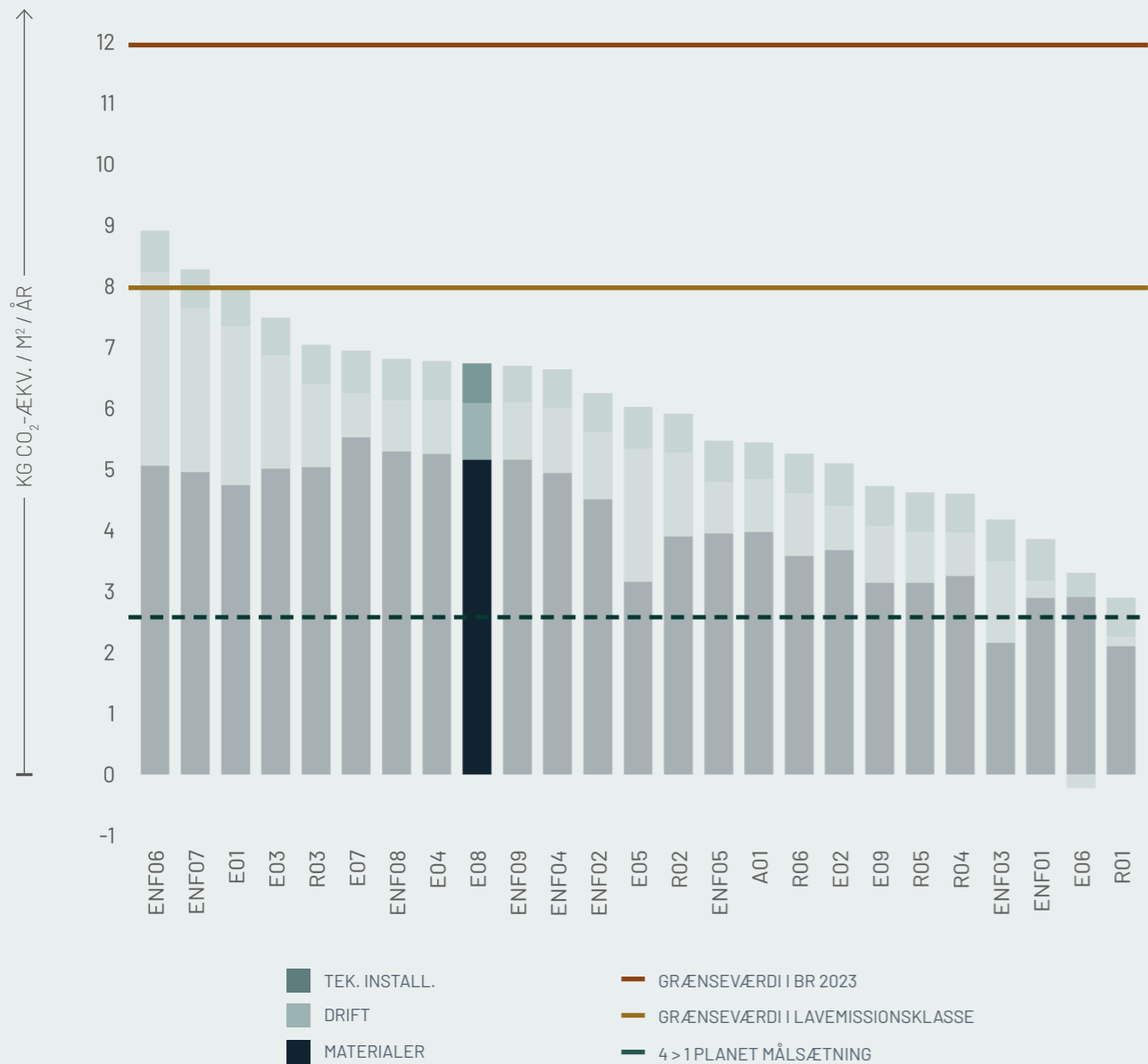
Figur E08.5: Boligcases Den vertikale akse viser udledning af kg CO 2 -ækv./m 2 /år. Den horisontale akse viser de 25 best practice cases.
