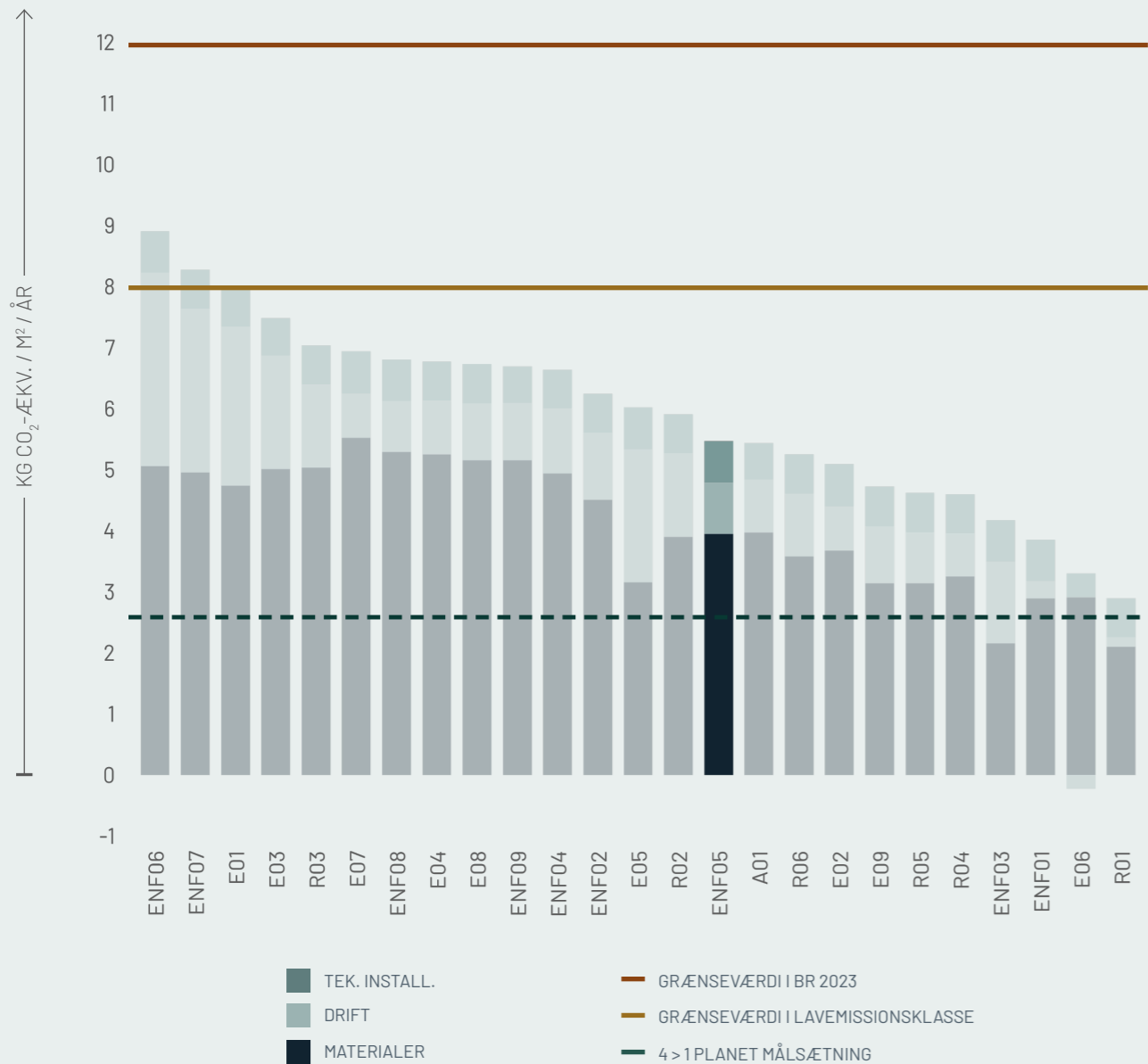
Figur ENF05.5: Boligcases Den vertikale akse viser udledning af kg CO 2 -ækv. / m 2 / år. Den horisontale akse viser de 25 best practice cases.
