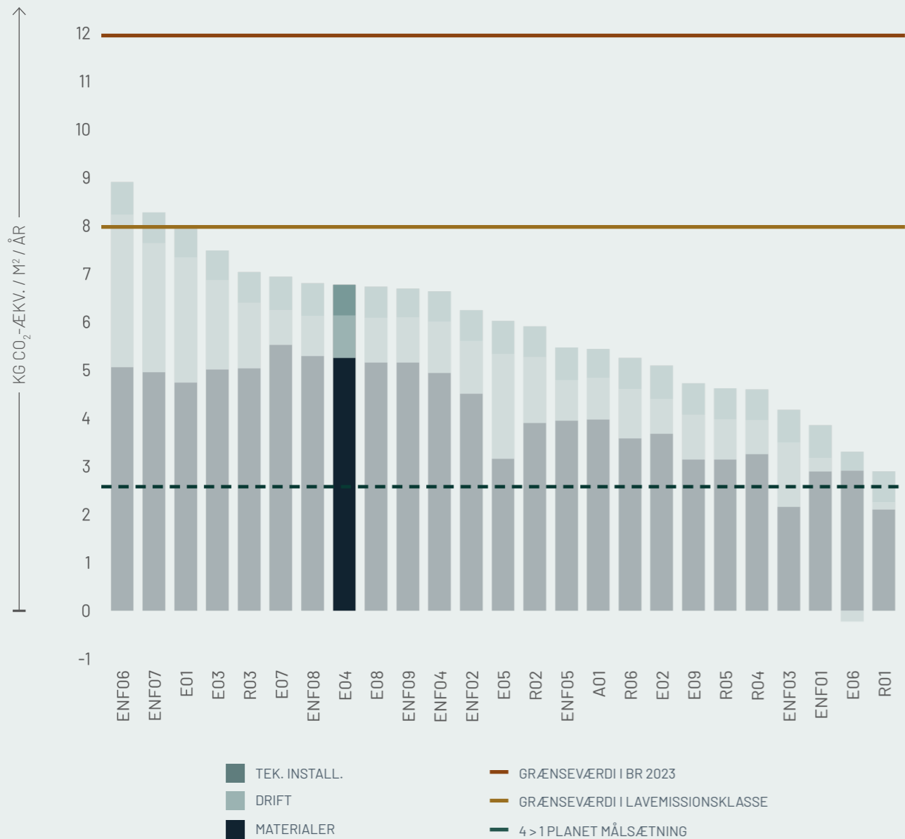
Figur E04.5: Boligcases Den vertikale akse viser udledning af kg CO 2 -ækv./m 2 /år. Den horisontale akse viser de 25 best practice cases.
