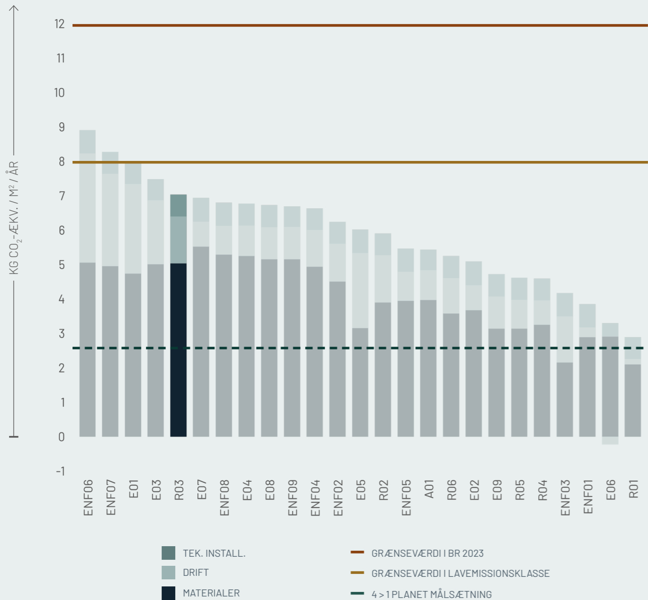
Figur E07.5: Boligcases Den vertikale akse viser udledning af kg CO 2 -ækv./m 2 /år. Den horisontale akse viser de 25 best practice cases.
