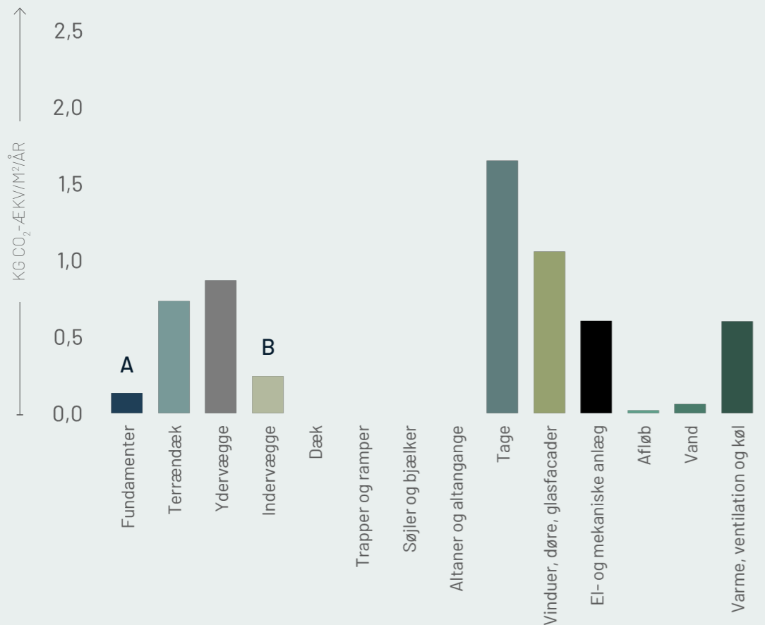
Figur ENF08.7: CO 2 -regnskab over byggeriets bygningsdele
