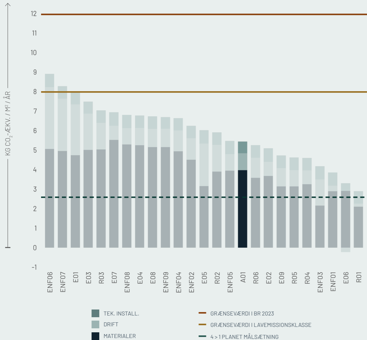
Figur A01.5: Boligcases Den vertikale akse viser udledning af kg CO 2 -ækv./m 2 /år. Den horisontale akse viser de 25 best practice cases.
