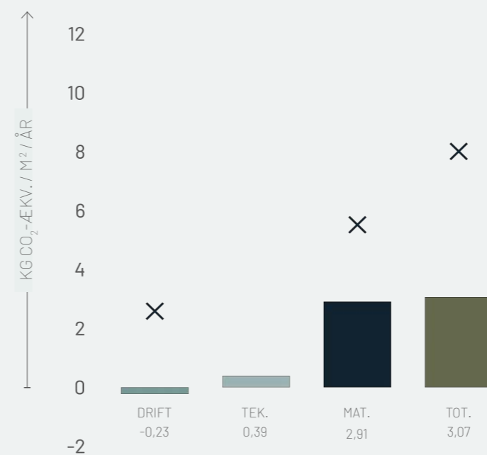
Figur E06.1: Udledningen af kg CO 2 -ækv. / m 2 / år Søjlerner viser bygningens klimapåvirkning. Krydsene indikerer det højeste resultat for drift, materialer og samlet udledning af kg CO 2 -ækv. / m 2 / år i casesamlingens etageboliger.
