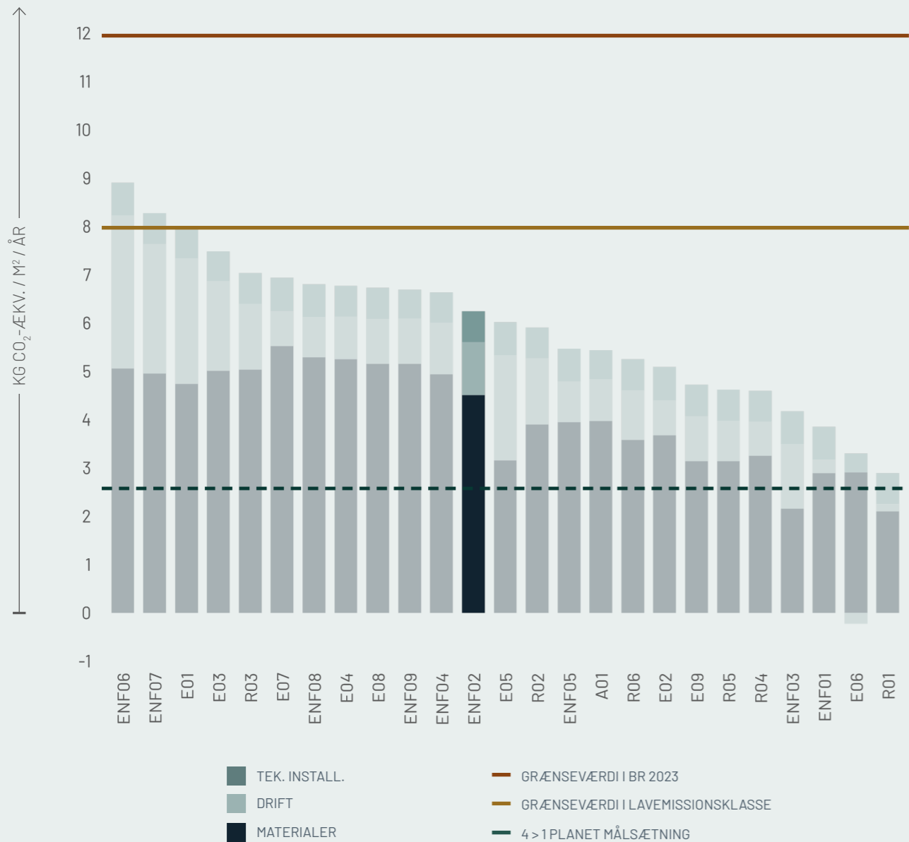
Figur ENF02.5: Boligcases Den vertikale akse viser udledning af kg CO 2 -ækv. / m 2 / år. Den horisontale akse viser de 25 best practice cases.
